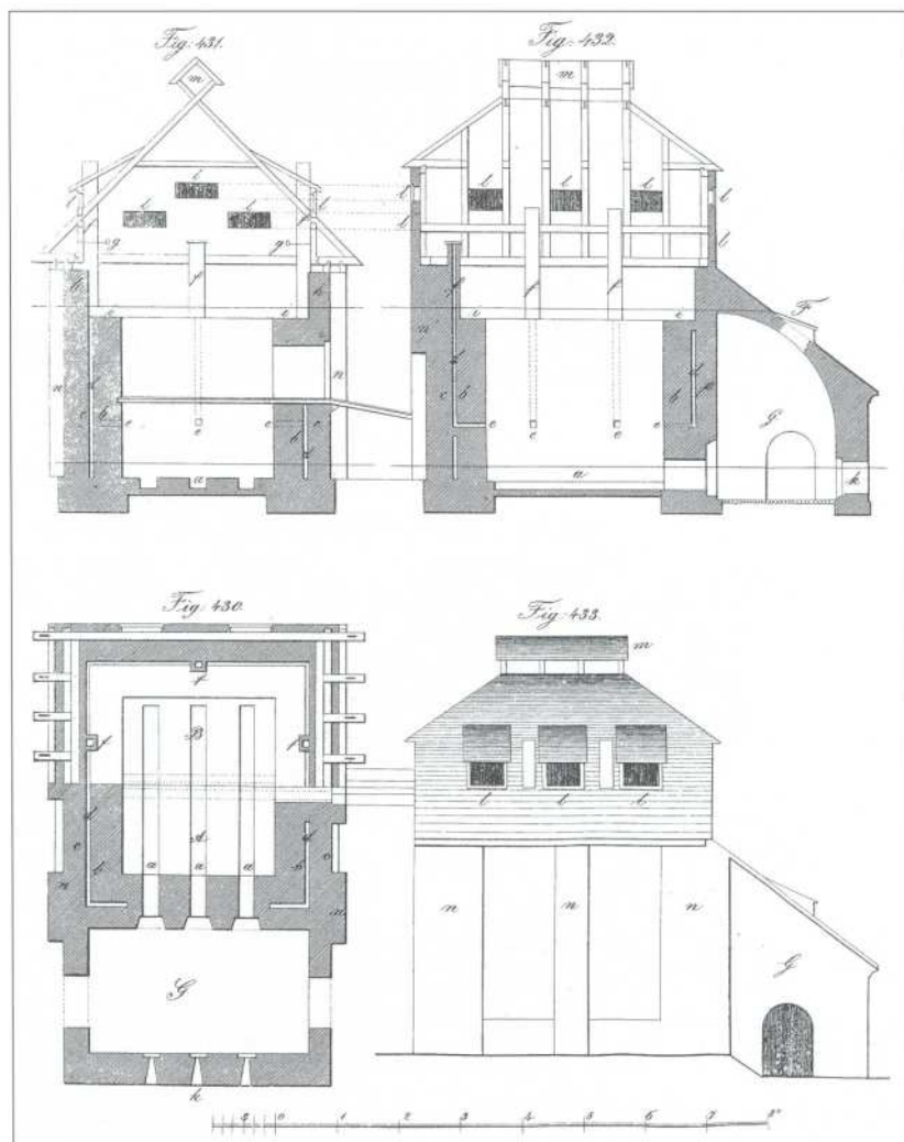
Vzorový typář pro stavbu cihlářských pecí z 1. třetiny 19. století (viz pozn. 7). Vysvětlivky některých popisek: a) popelník; b) obvodová stěna komory pece; G) předpeční komunikační prostor; l, m) přístřešek zakrývající pec s průduchy na odtah spalin; n) postranní nakládací otvor.
